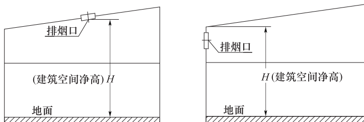
图 A-3 斜坡屋顶示意图
