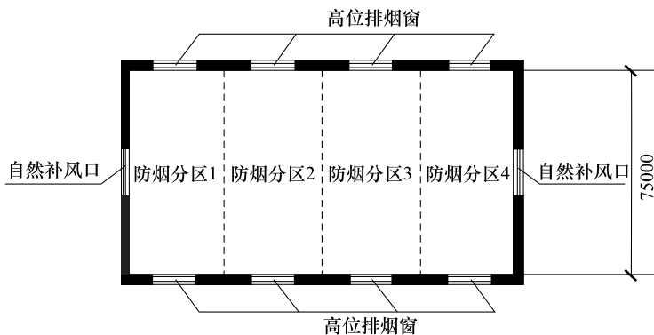
图5.2.3 具备对流条件场所自然排烟窗的布置示意
