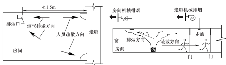
图 5.4.8 排烟口设置示意图
