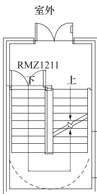
(a) 地上地下楼梯间共用
