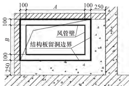
图 B-6 风井内结构楼板留洞尺寸图
