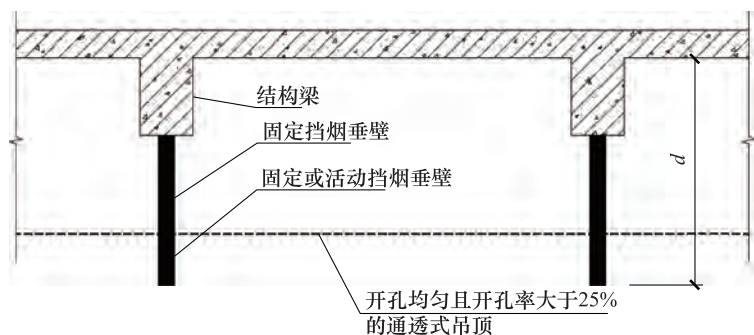
图 5.6.2-2 开孔均匀且开孔率大于 25% 的通透式吊顶挡烟垂壁设置及储烟仓厚度 ( d ) 示意图
