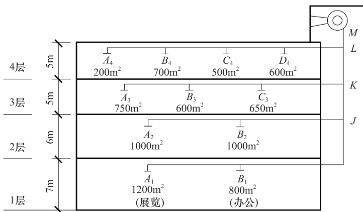
图 5.6.6 排烟系统示意图
