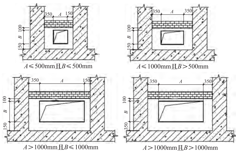
图 B-3 一面后砌墙风管安装尺寸
