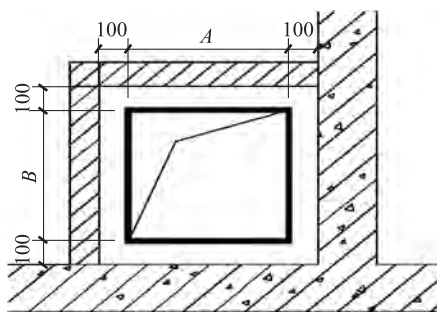
图 B-5 吊装风管安装尺寸（楼板留洞同风井尺寸）
