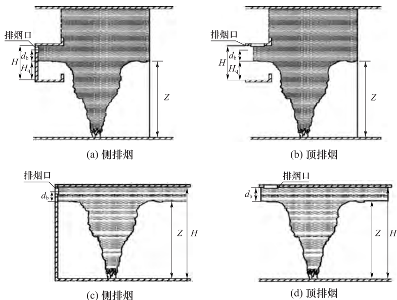
图 5.6.17 排烟口设置位置参考图
