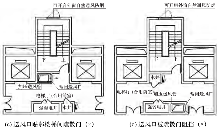
图 4.1.4 防烟楼梯间自然通风，前室加压送风口设置示意图
