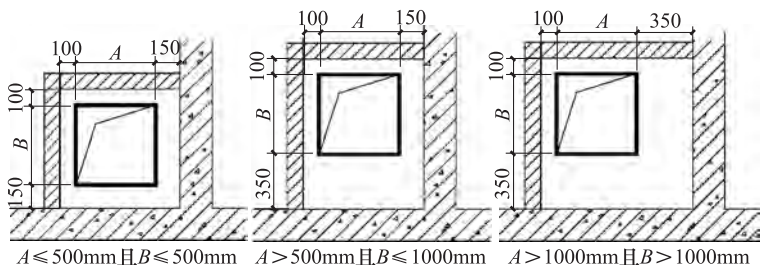
图 B-2 两面后砌墙风管安装尺寸
