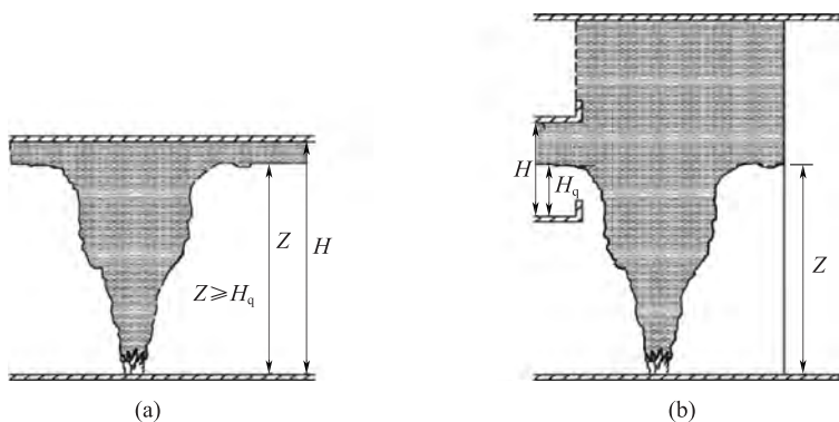
图 5.6.11-1 最小清晰高度示意图
