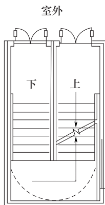
(b) 地上地下楼梯间不共用
