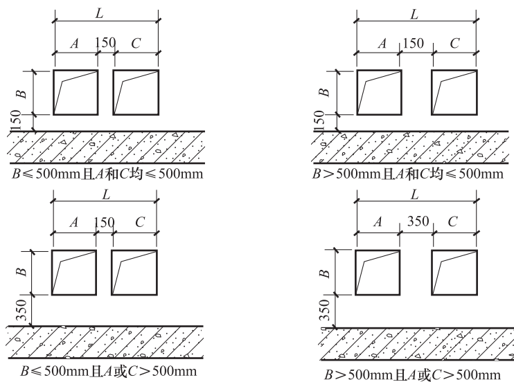
图 B-4 两个及以上风管并排安装时的安装尺寸
