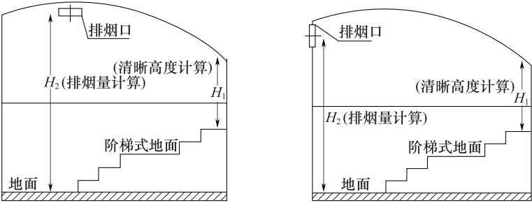
图 A-6 斜屋顶、阶梯式地面的场所示意图
