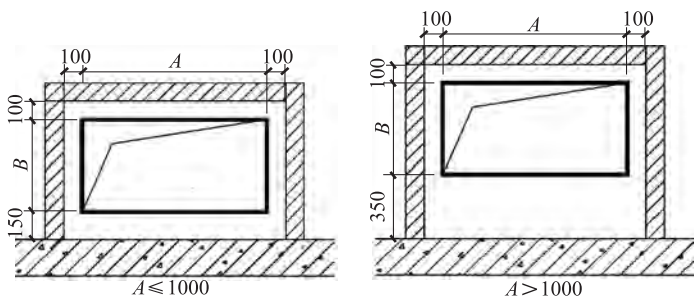
图 B-1 三面后砌墙风管安装尺寸
