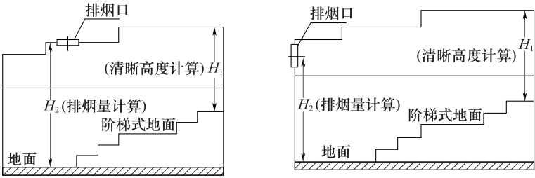
图 A-5 阶梯叠级式屋顶、阶梯式地面的场所示意图
