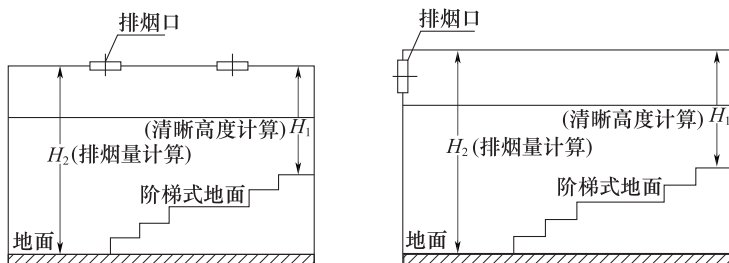
图 A-4 平屋顶面、阶梯式地面的场所示意图
