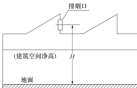
图 A-1 锯齿形屋顶示意图
